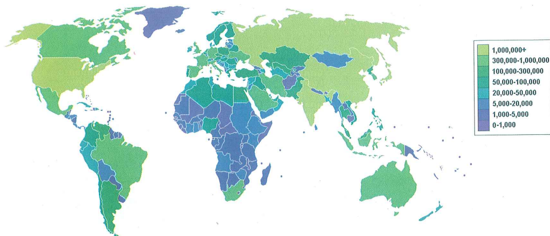
Emisión de dióxido de carbono, por país, en millones de toneladas.
